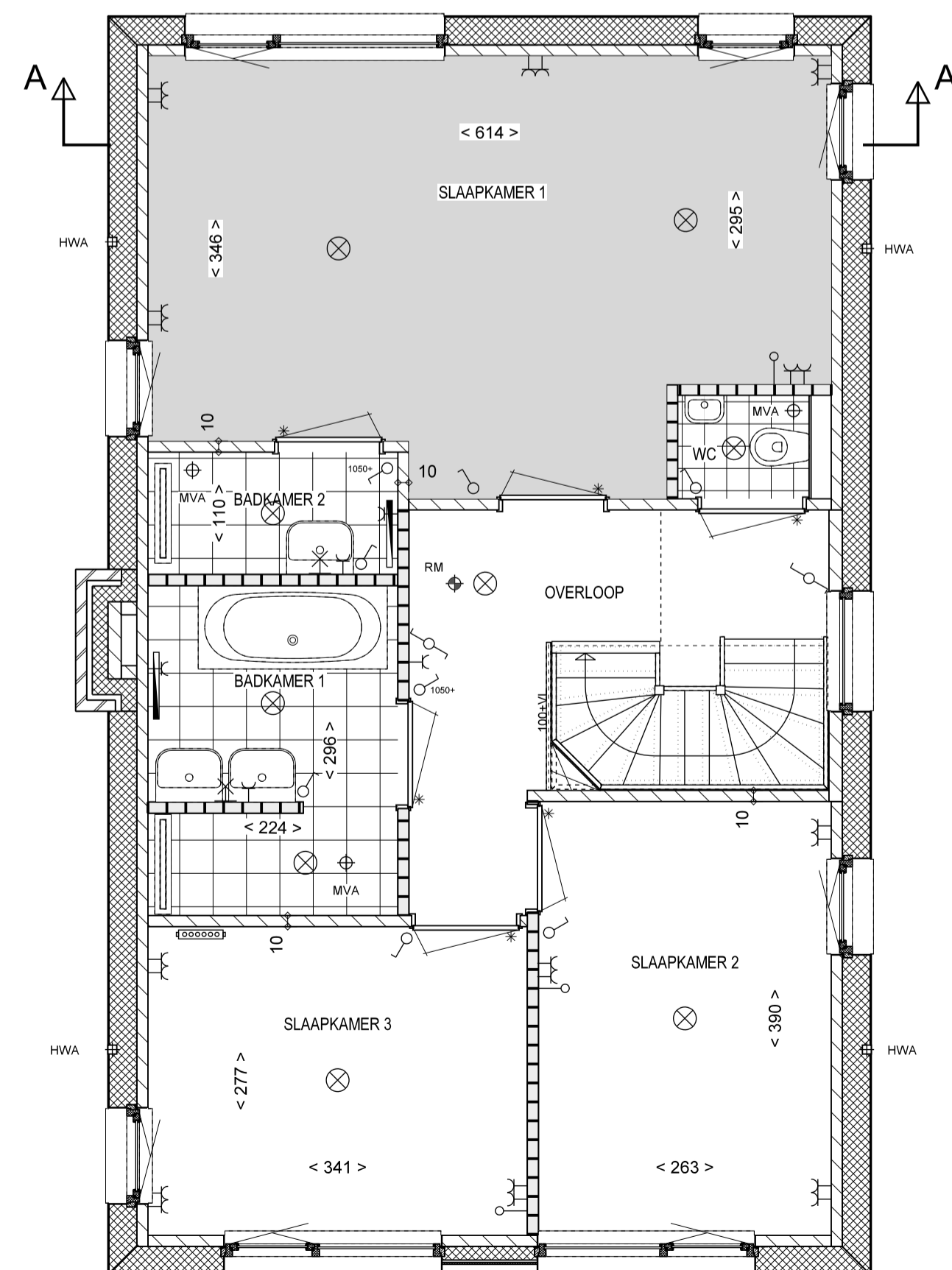
OPTIE 7: 3 SLAAPKAMERS, 2 BADKAMERS, MASTERBEDR ACHTER 1e VERDIEPING
