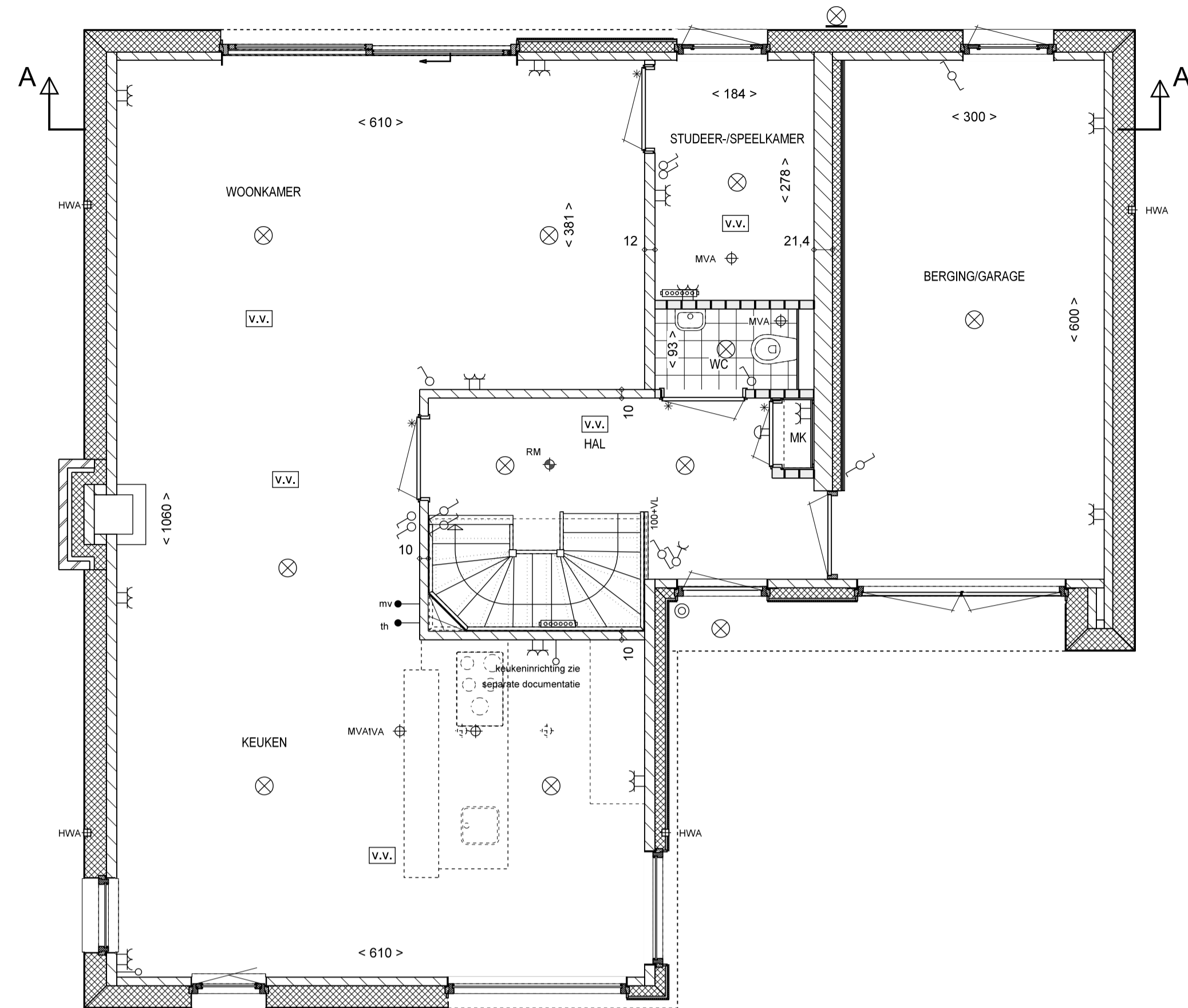
OPTIE 5: KEUKEN VOORZIJD, WOONKAMER ACHTER BEGANE GROND
