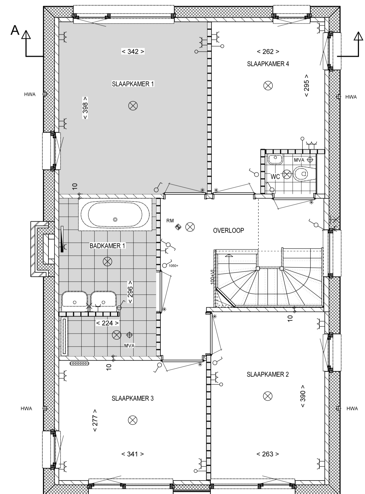
OPTIE 8: 4 SLAAPKAMERS EN 1 BADKAMER 1e VERDIEPING
