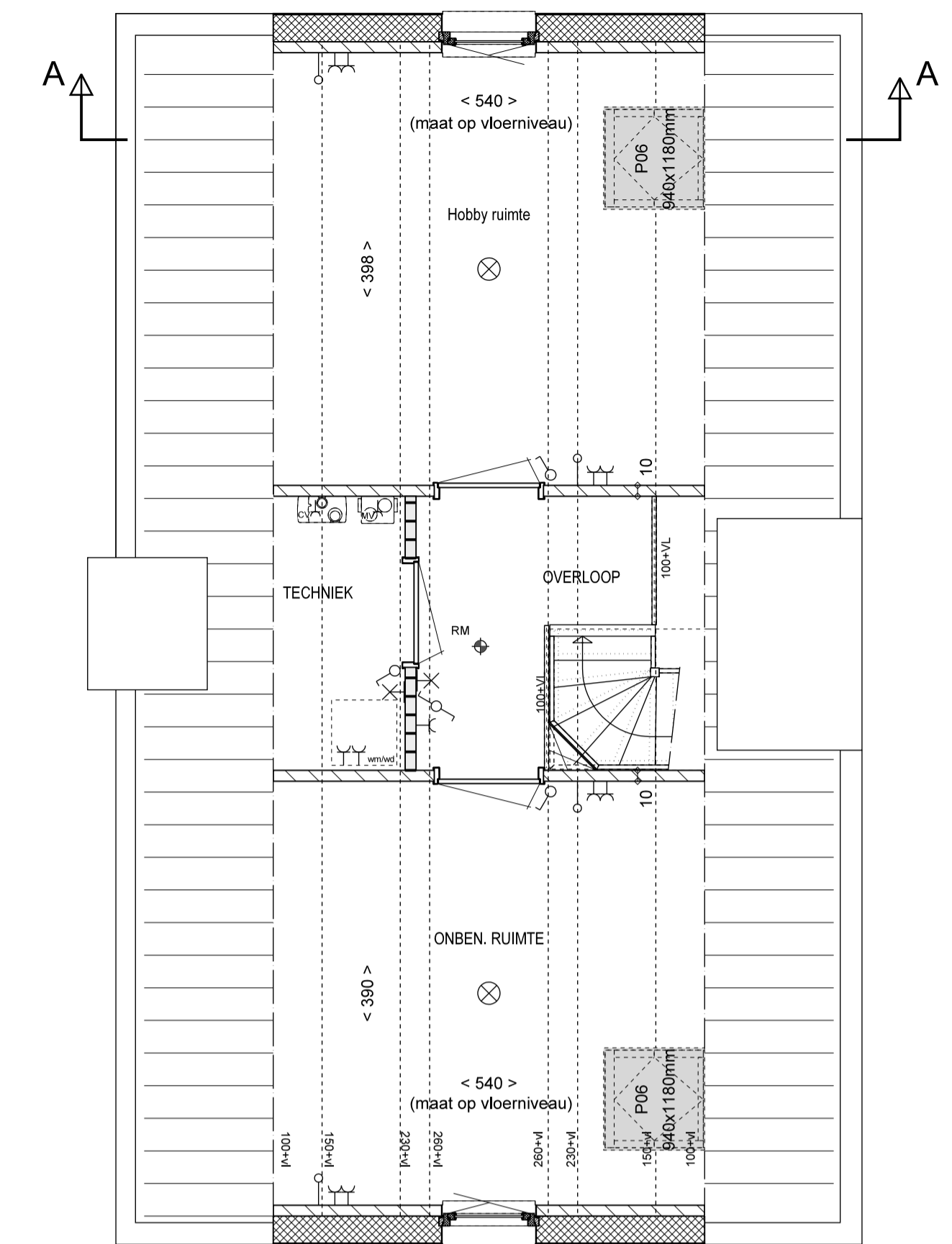
OPTIE 9: DAKRAMEN OP ZOLDER 2e VERDIEPING
