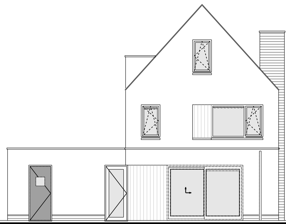
KAVEL 10, KAVEL 3 GESP. OPTIE 1: UITBOUW 120cm ACHTERGEVEL
