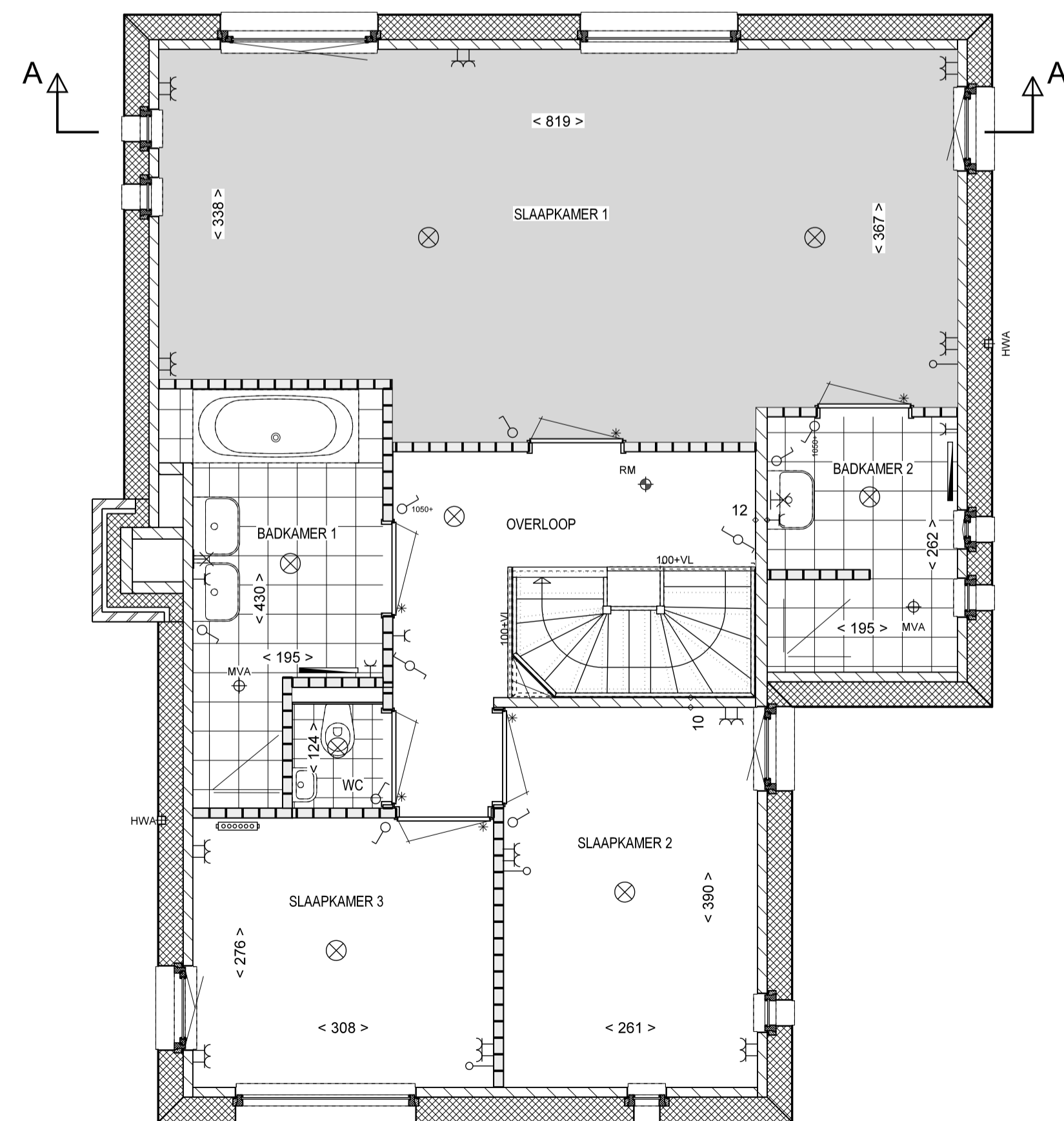
OPTIE 7: 3 SLAAPKAMERS, 2 BADKAMERS, MASTERBEDR. ACHTER 1e VERDIEPING
