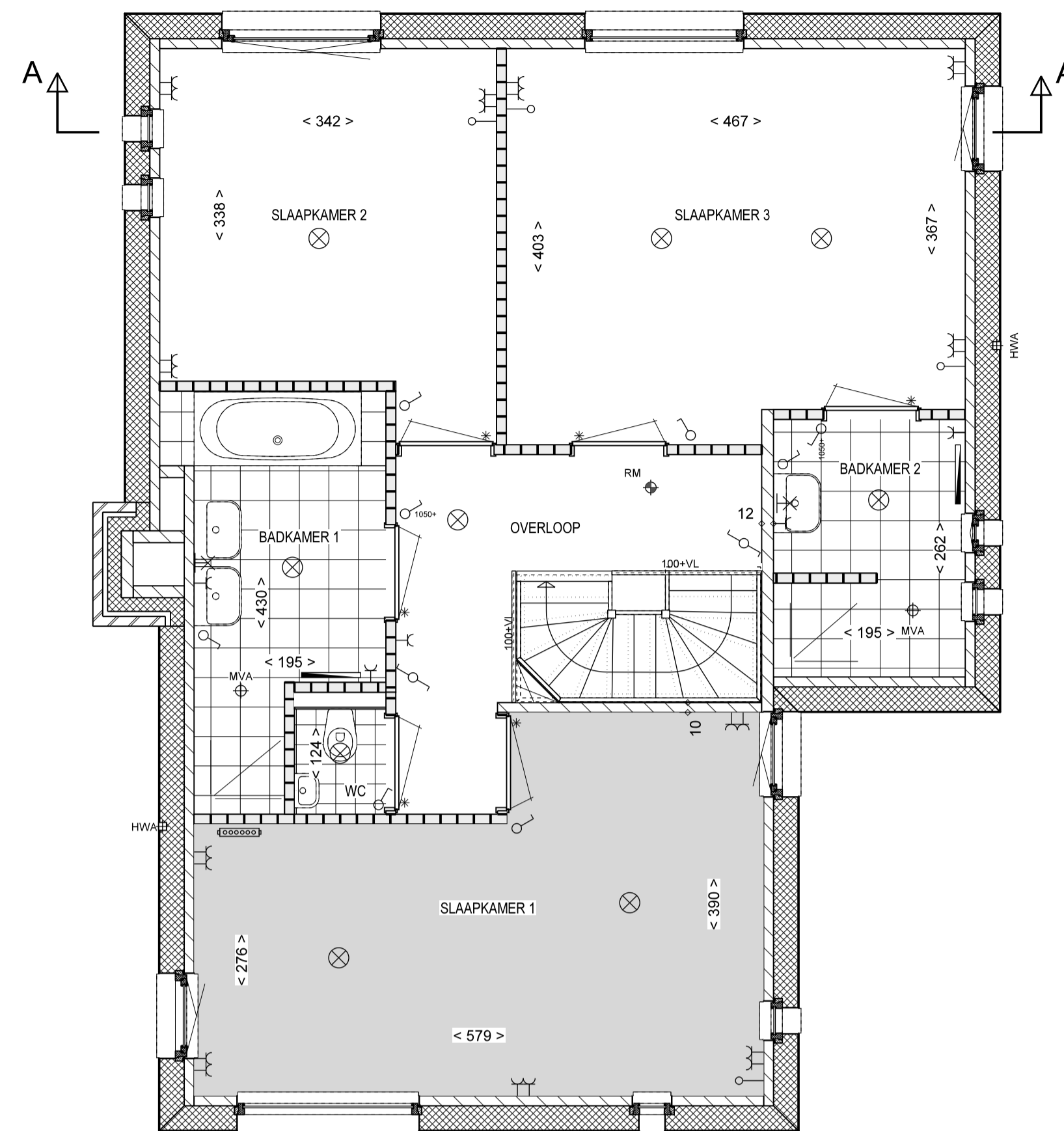
OPTIE 6: 3 SLAAPKAMERS, 2 BADKAMERS, MASTERBEDR. VOOR 1e VERDIEPING
