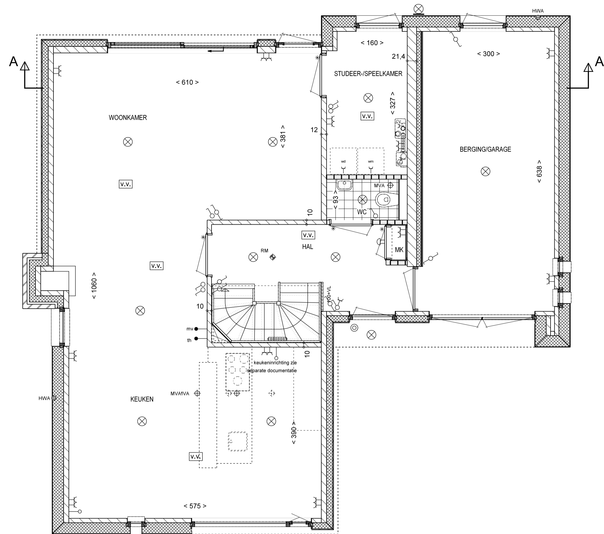
OPTIE 5: KEUKEN VOORZIJD, WOONKAMER ACHTER BEGANE GROND
