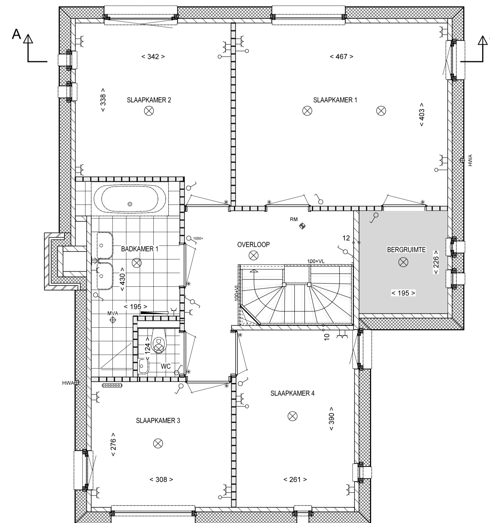
OPTIE 8: 4 SLAAPKAMERS EN 1 BADKAMER 1e VERDIEPING
